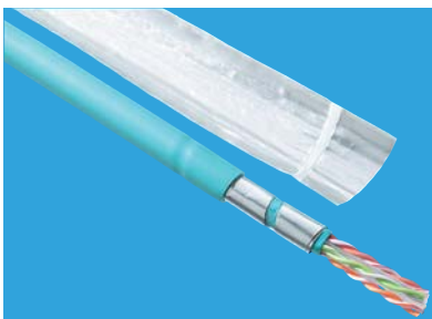
Кабель R&M: наличие отрезков фольги устраняет перекрестные помехи.
