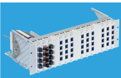
Панель Global: держатели устанавливаются вертикально. Можно разместить голосовые модули, коаксиальные разъемы, оптические модули прямого терминирования, а также модули с кассетой для сплайсов.
