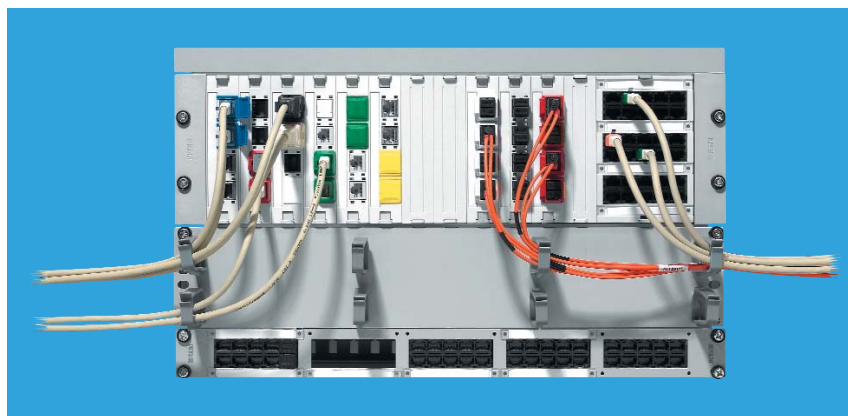
Коммутационная панель Global: в одно и то же изделие можно устанавливать модели разъемов как для медных, так и для оптических трактов.
