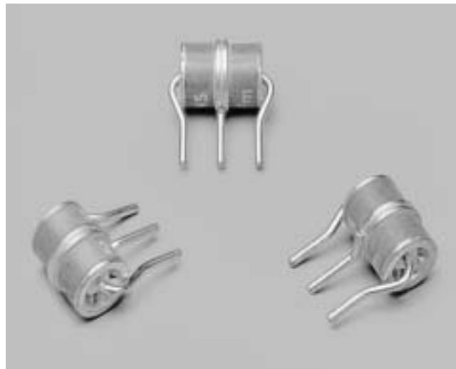
3-электродный разрядник без элемента термозащиты Fail-safe.
